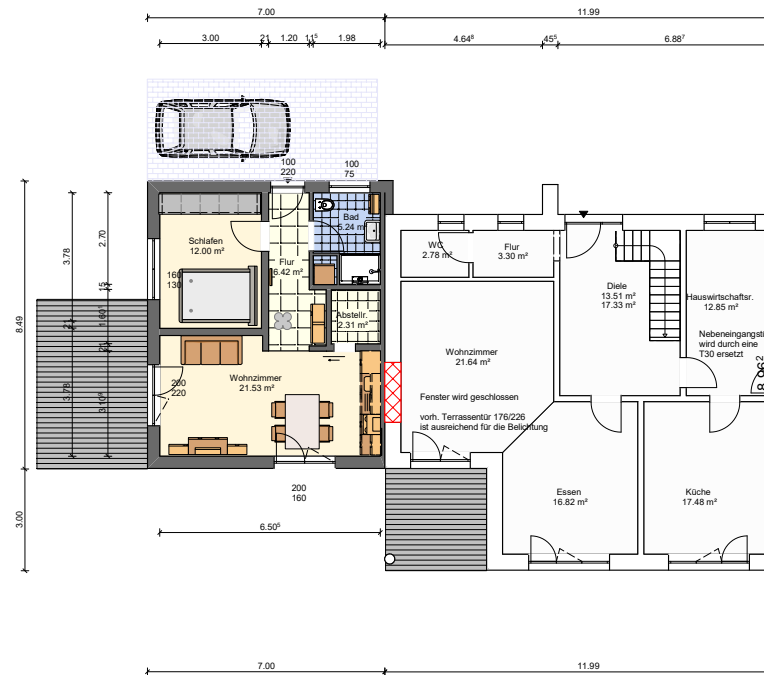
geplante Einliegerwohnung -vormals Garten-
